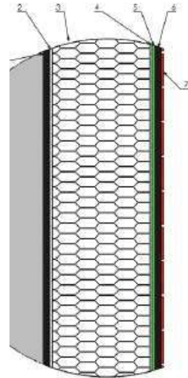
Sección constructiva de panel de aislamiento en baños de vapor
